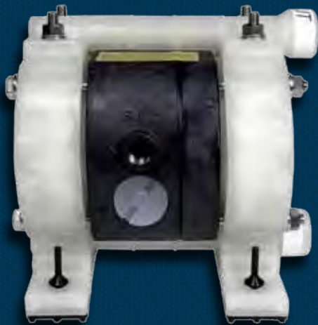
Насос NDP-5 Полипропилен Габариты: 156 мм x 152 мм Вес нетто: 1,36 кг Вес брутто: 1,81 кг
